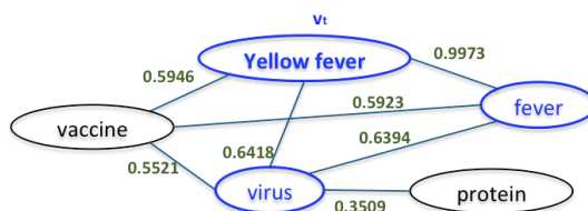
Figure 3. Sous-graphe créé pour le terme Yellow Fever
